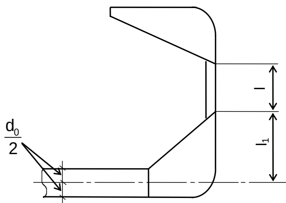
Hình 2A/29.2 Xác định h, l_1
