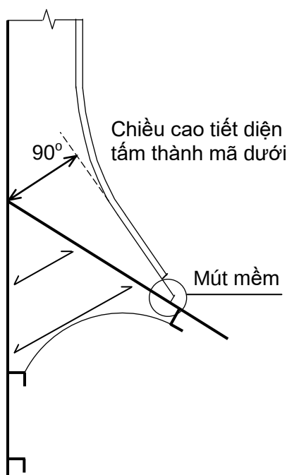
Hình 2A/29.15 Xác định chiều cao tiết diện tấm thành mã dưới khi tính t_{REN,dft}
