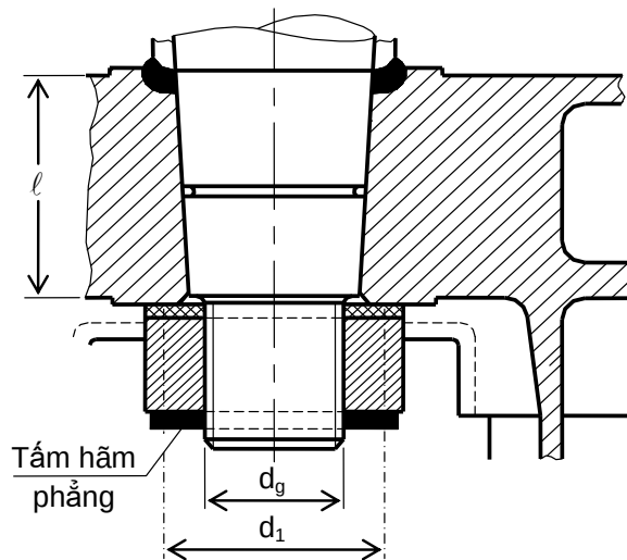
Hình 2A/25.8 Mối nối côn không then
