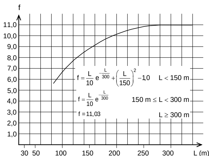
Hình 2A/16.1 Trị số của f
