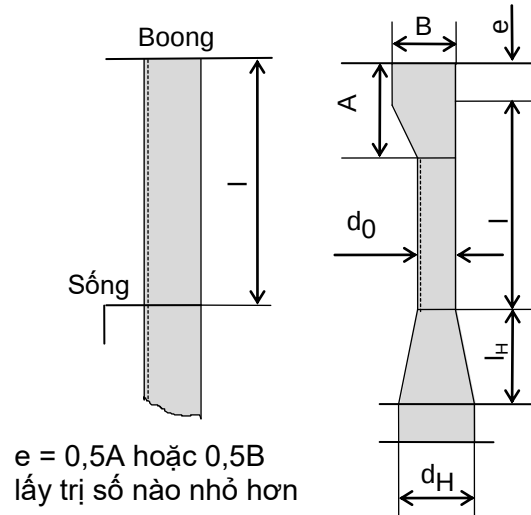
Hình 2A/11.3 Đo l
