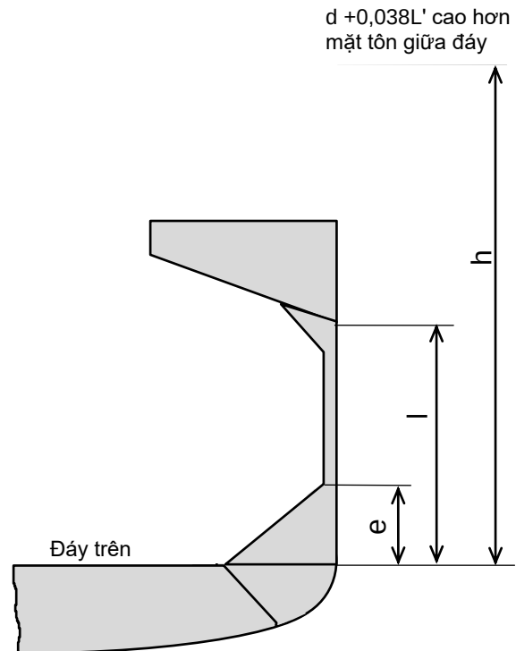
(b) Hệ thống kết cấu có kết đỉnh mạn
