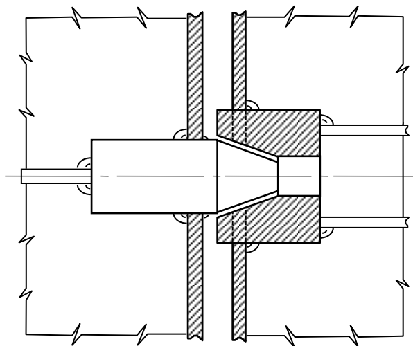
Hình 2B/19.4 Ổ chặn
