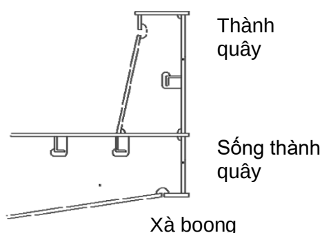
Hình 2B/17.9 Sự kéo dài của tấm thành quây
