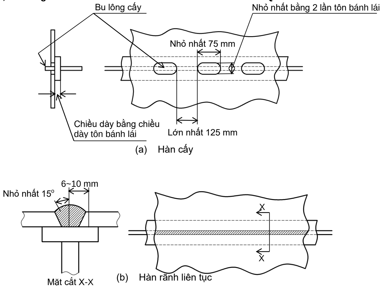
Hình 2B/21.1.2 Hàn cấy và hàn rãnh liên tục
