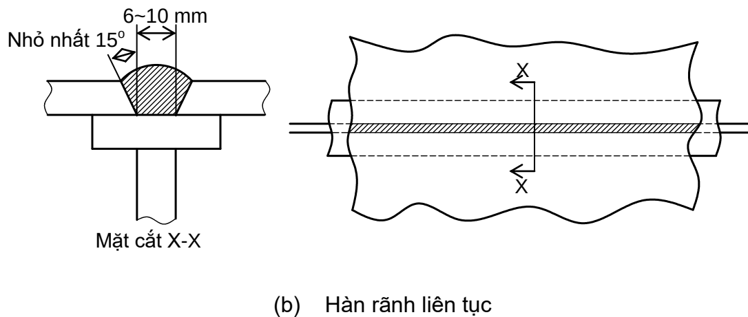
Hình 2A/25.2 Hàn cây và hàn rãnh liên tục
