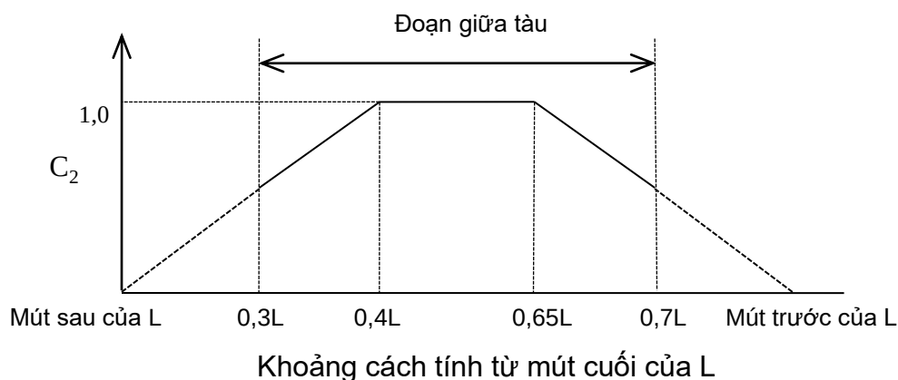
Hình 2B/13.1 Trị số của hệ số C_2
