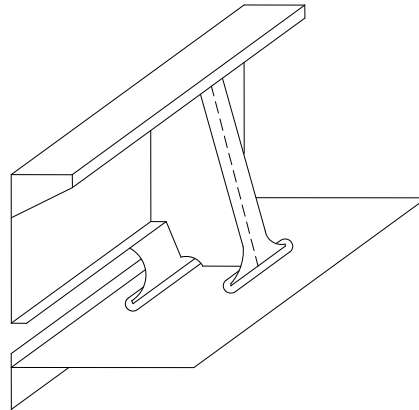
Hình 2A/21.2 Kiểu có tấm đệm
