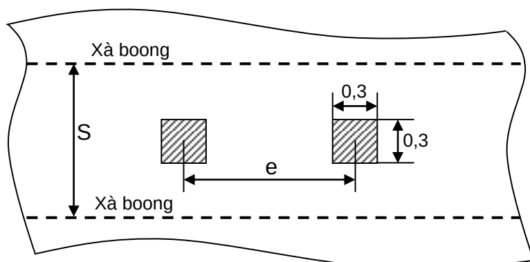
Hình 2A/10.3 Khoảng cách đo e
