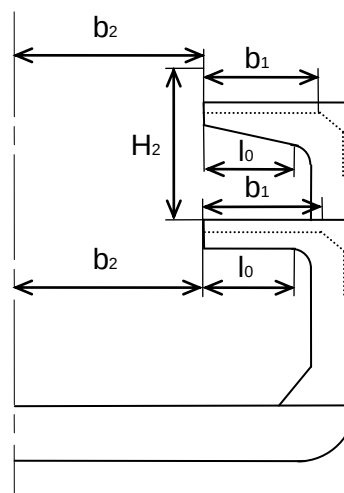
Đo l_0 , b_1 , b_2 và H_2
